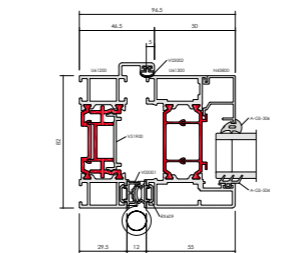
F82 Jamb
