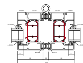
F82 Interlock
