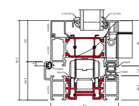
F82 Cill
