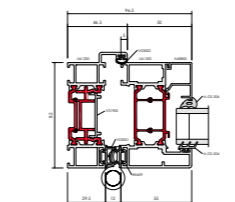
F82 Jamb
