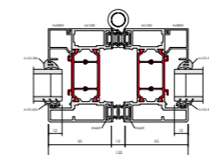
F82 Interlock
