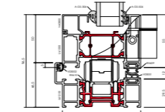
F82 Cill
